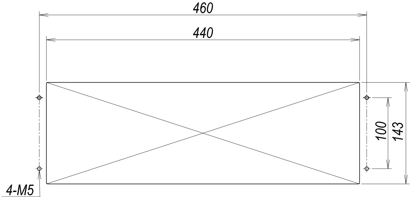
パネルカット図
